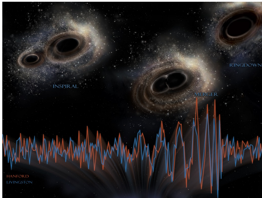
Vue d'artiste montrant trois étapes de la fusion des deux trous noirs de l'événement GW150914 ainsi que les signaux (courbes rouge et bleue ; durée : environ trois dixièmes de seconde) enregistrés par les deux détecteurs LIGO Avancés. Ils ont été superposés pour mieux faire ressortir leurs ressemblances © LIGO/Aurore Simonnet
